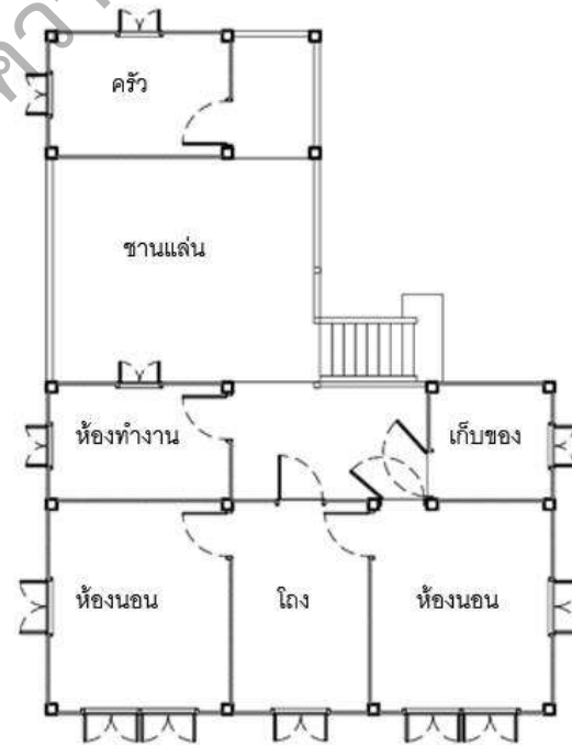
ผังพื้นที่ชั้นบน
