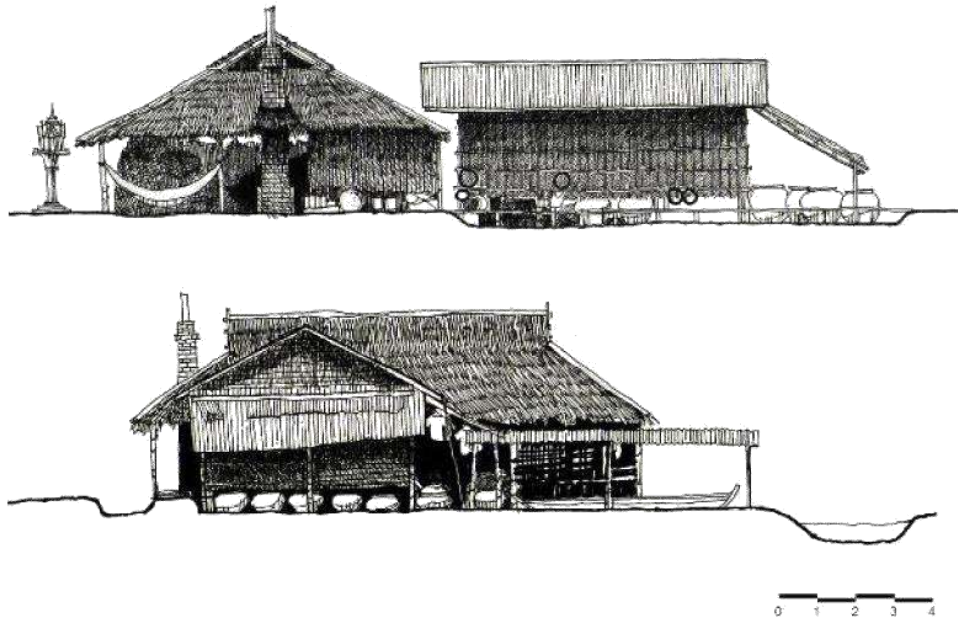
บน: รูปด้านหน้าเรือนพื้นถิ่นชาวสวนมะพร้าวกรณีศึกษา ล่าง: รูปด้านข้างเรือนพื้นถิ่นชาวสวนมะพร้าวกรณีศึกษา
